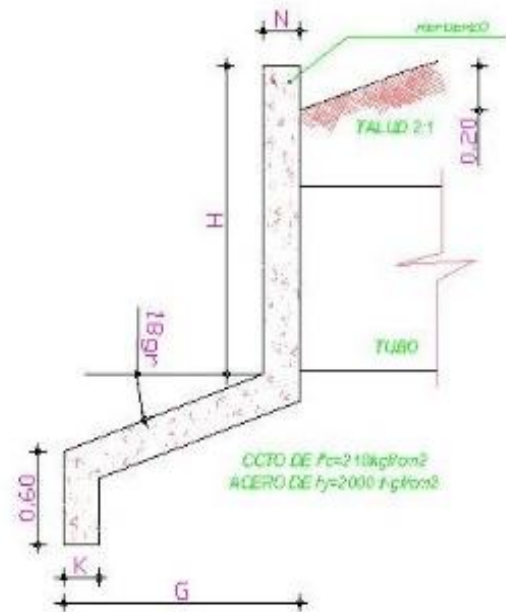
SECCION A-A
